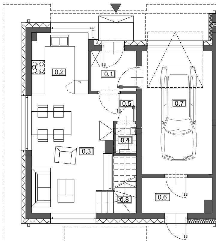
RZUT PARTERU
