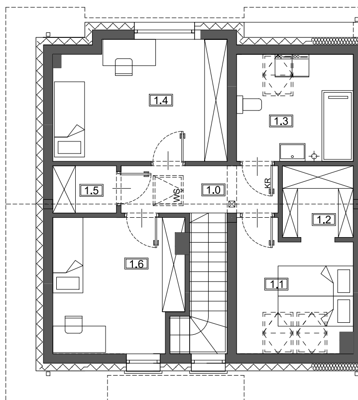
RZUT PODDASZA
